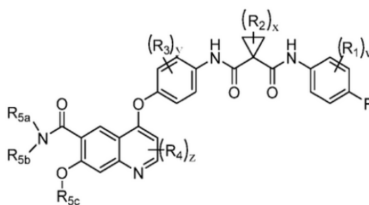
Formulė I
