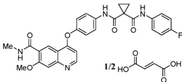
Junginys 1-hemifumaratas
