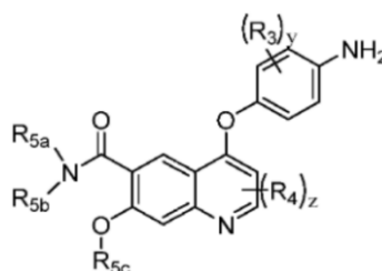
Formulė II
