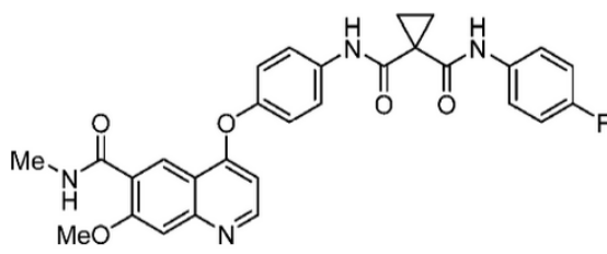
Junginys 1
