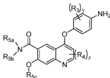
Formulė II
