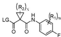
Formulė III
