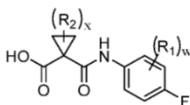
Formulė IV
