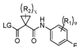
Formulė III
