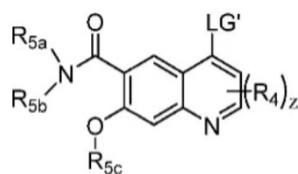
Formulė V
